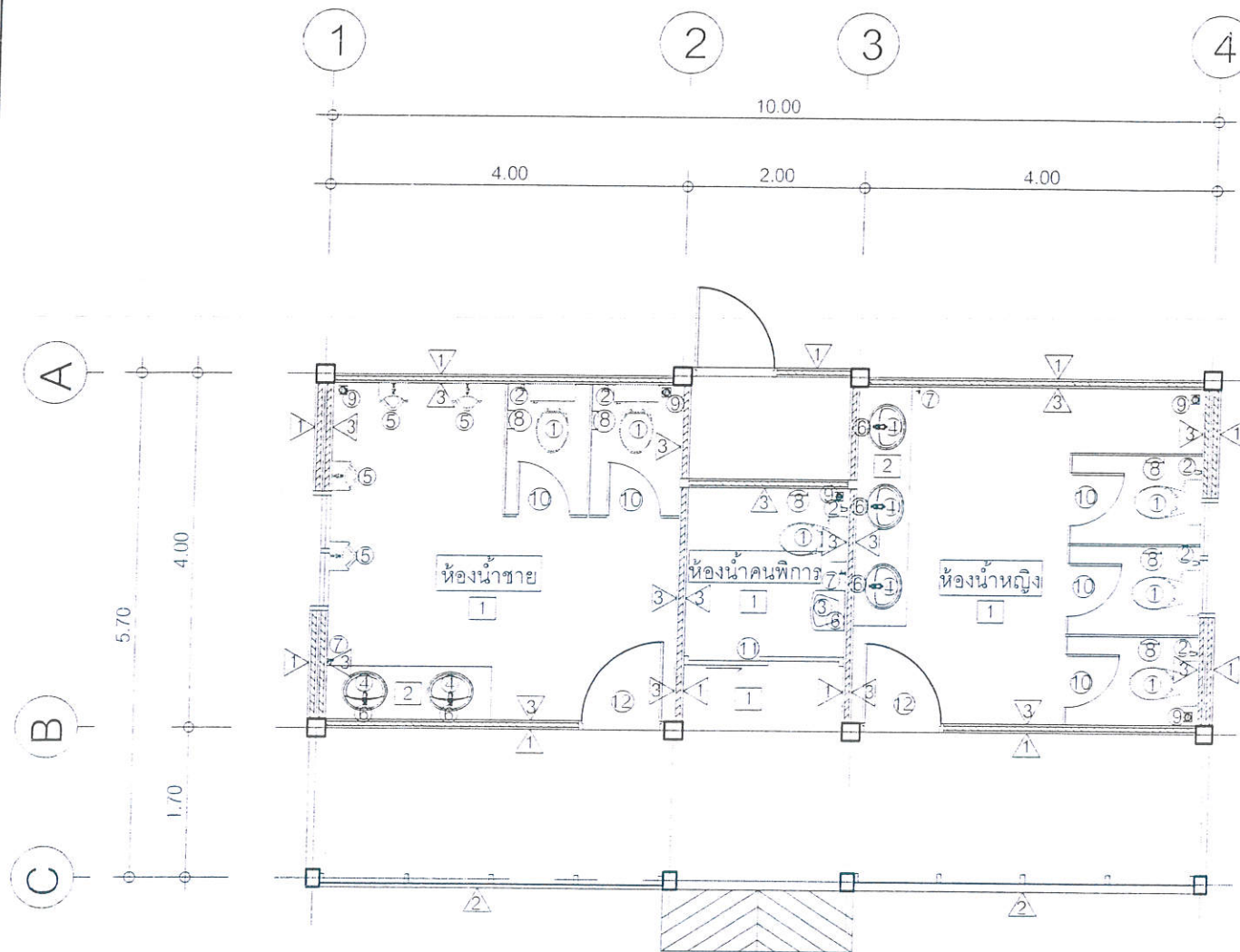
แปลนพื้นห้องน้ำ (ปรับปรุง) SCALE 1:75
