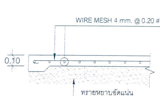
ขยาย GS SCALE 1:20
